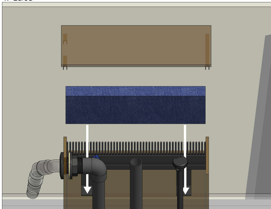
Schéma 4 : Trop-plein avec éponge et couverture
