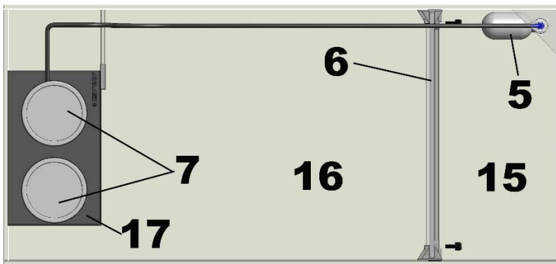
Fig. 1: Sumidero de filtro Armatus Lagoon 400
